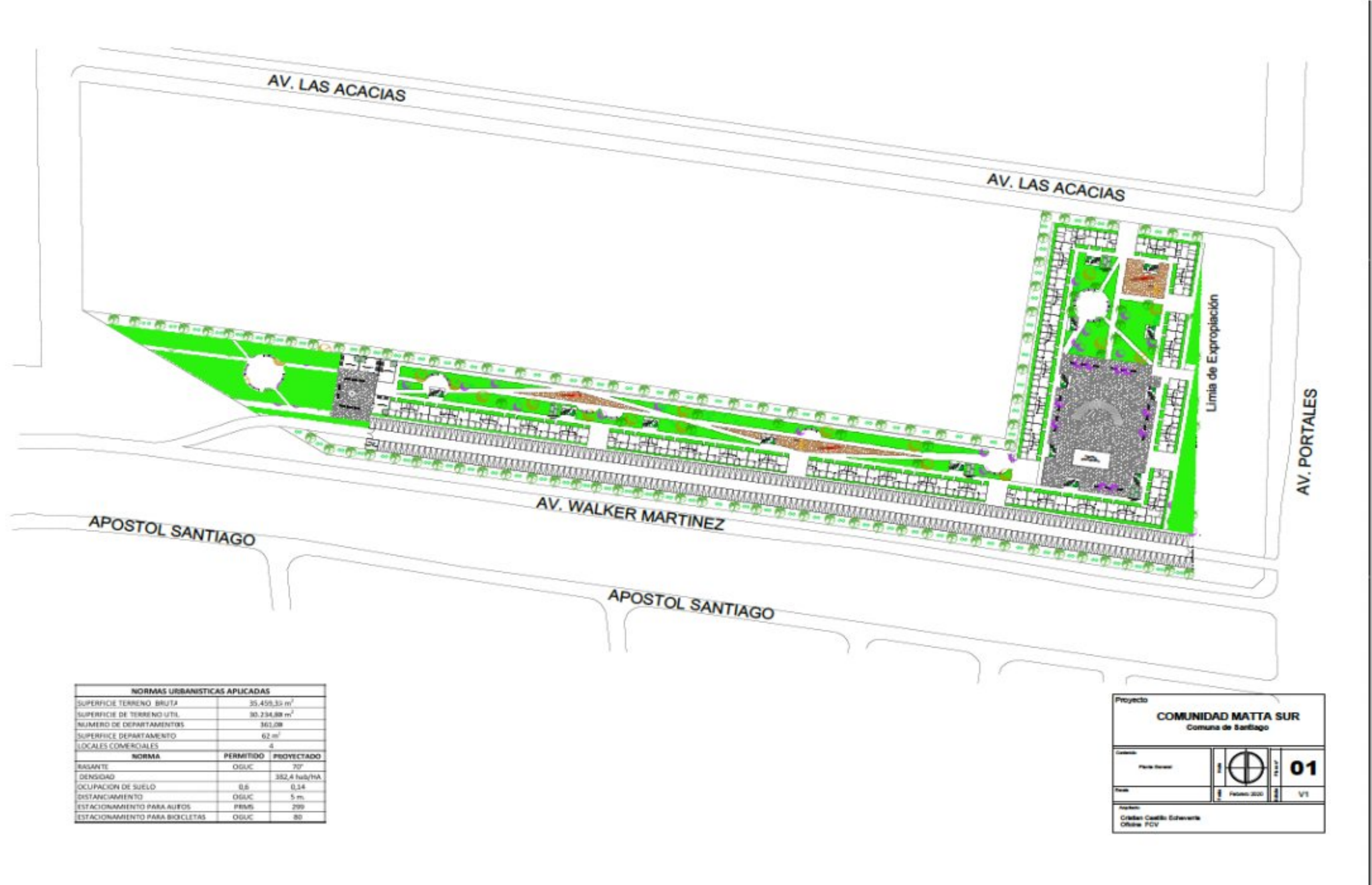
Imagen N°2: Mapa del anteproyecto para la construcción de viviendas sociales en inmueble antes individualizado, confeccionado por el arquitecto Sr. Cristian Castillo Echeverría.
